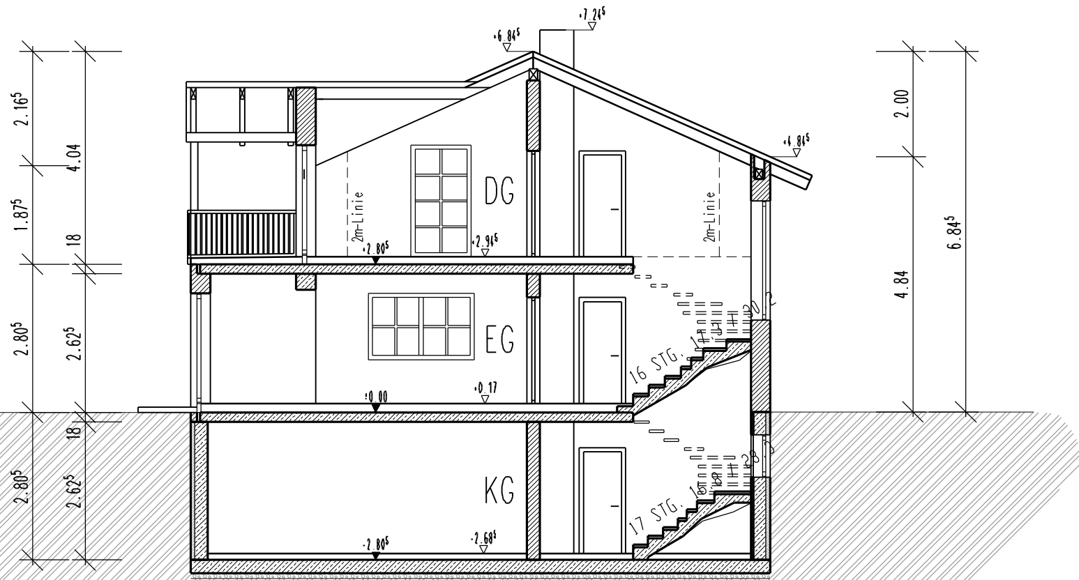
Schnitt A-A
